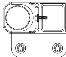
Schnitt B-B
