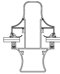
Träger Art.-Nr.: 1235
