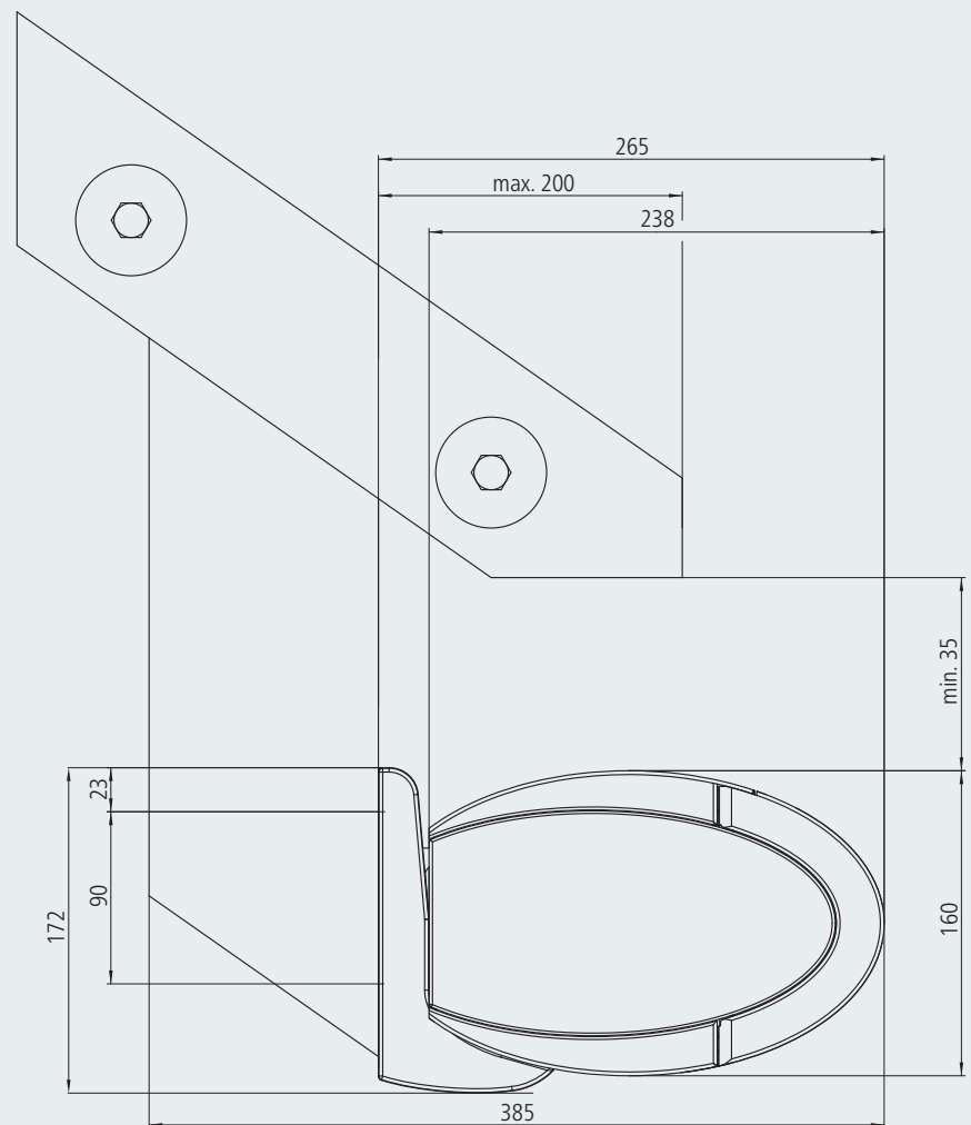
Seitenansicht Dachsparrenmontage
